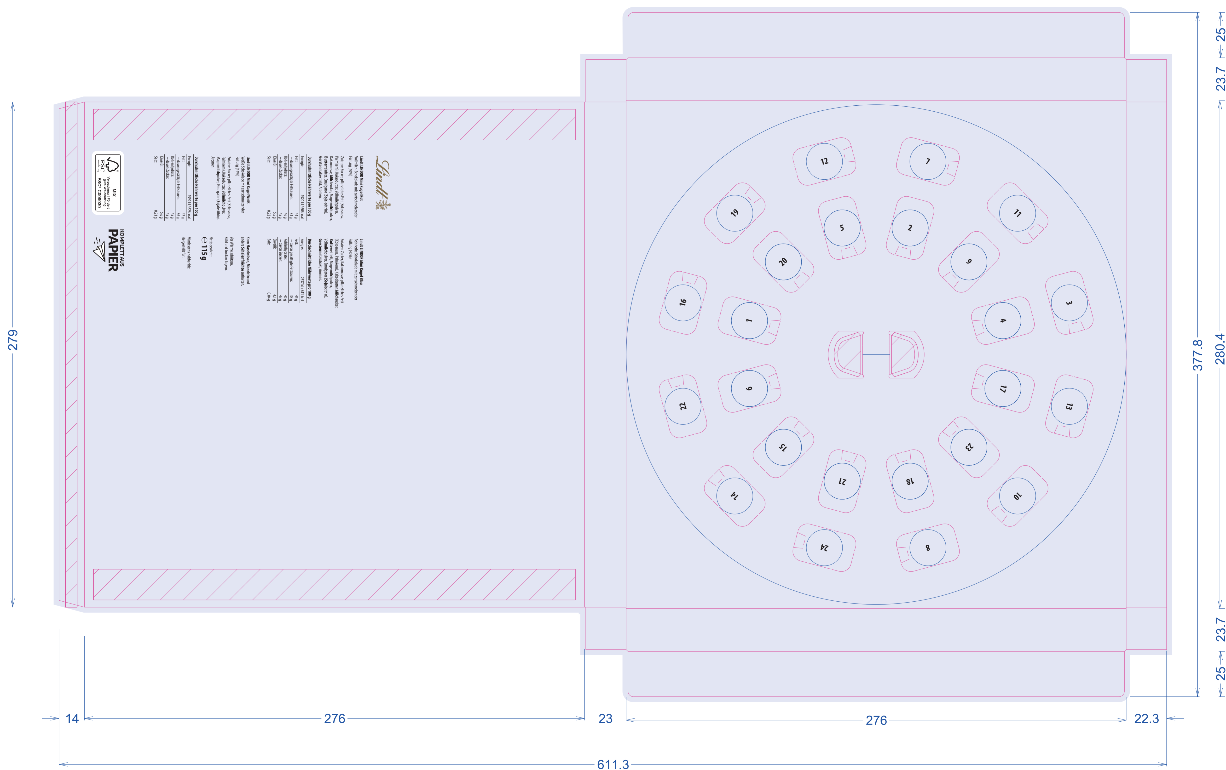
Fixierplatte
